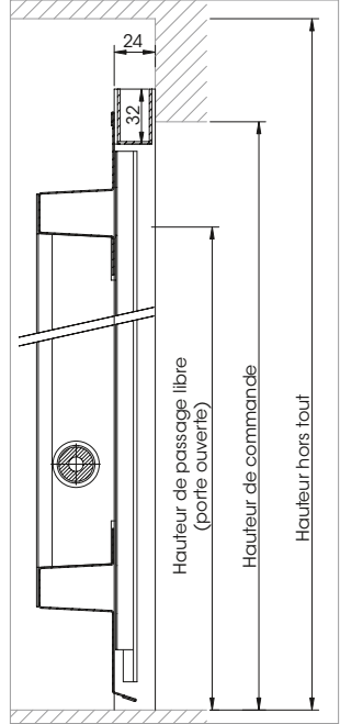
Coupe verticale
