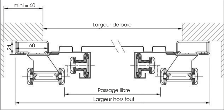
Coupe horizontale
