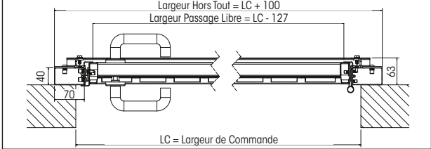
Bâti d'angle
