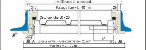
Bâti tubulaire
