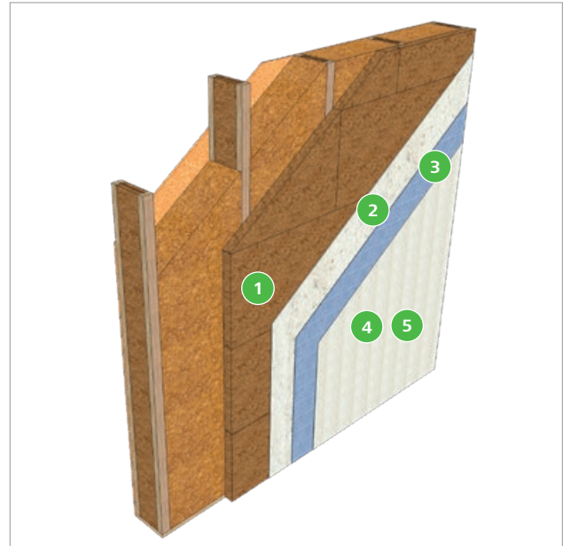
Ossature bois avec contreventement intérieur
