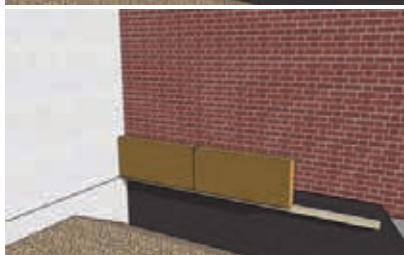
Encoller le panneau par un boudin périphérique au dos de celui-ci et deux plots au droit des fixations.
